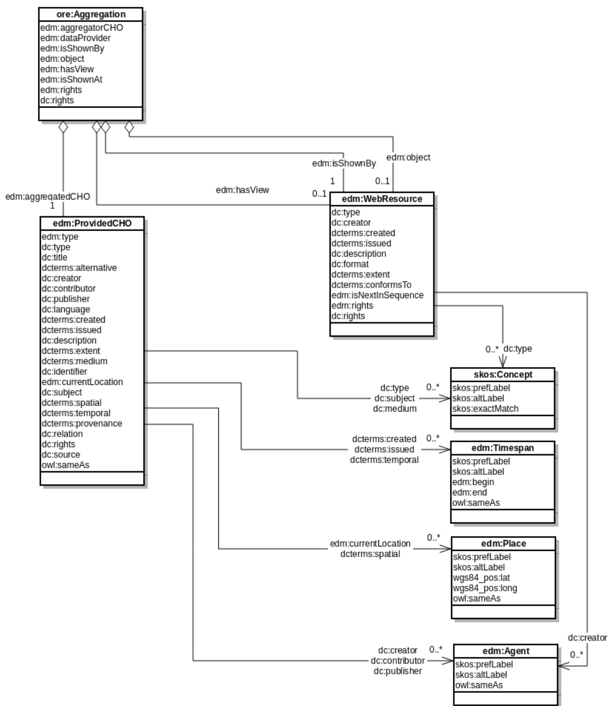
Εικόνα 2. Διάγραμμα κλάσεων του EDM μοντέλου
