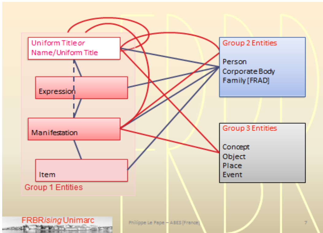
Σχ. 4: FRBR: Σχέσεις μεταξύ των τριών ομάδων κλάσεων από το Σεμινάριο του Philippe Le Pape “FRBRising Unimarc” [16]
