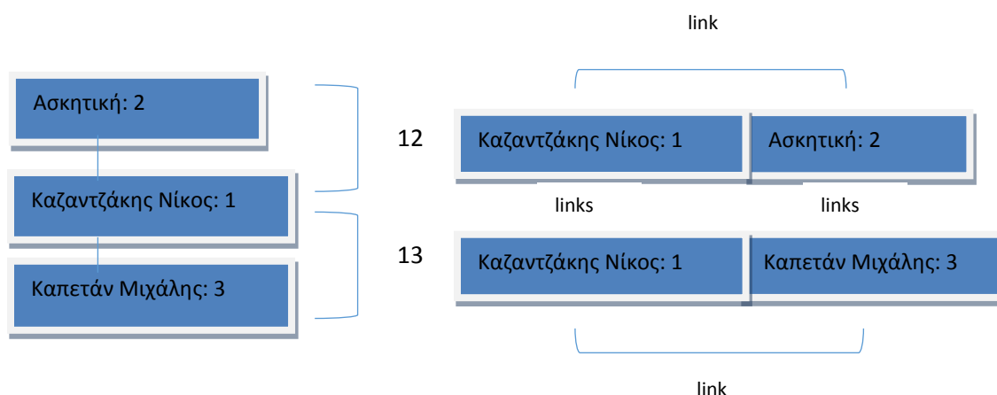
Σχ. 6: Embedded τεχνική για την οντότητα Ονομα/Τίτλος
