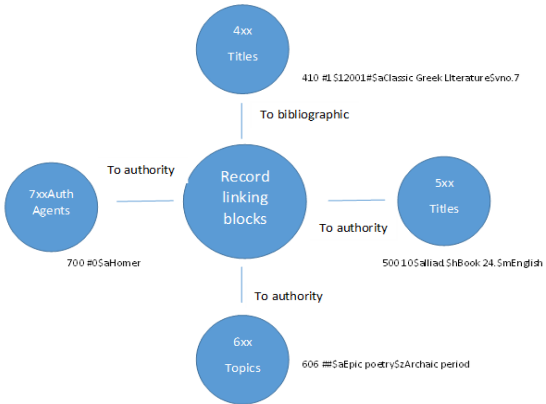
Σχ. 1: UNIMARC: Οι διασυνδέσεις της βιβλιογραφικής οντότητας
