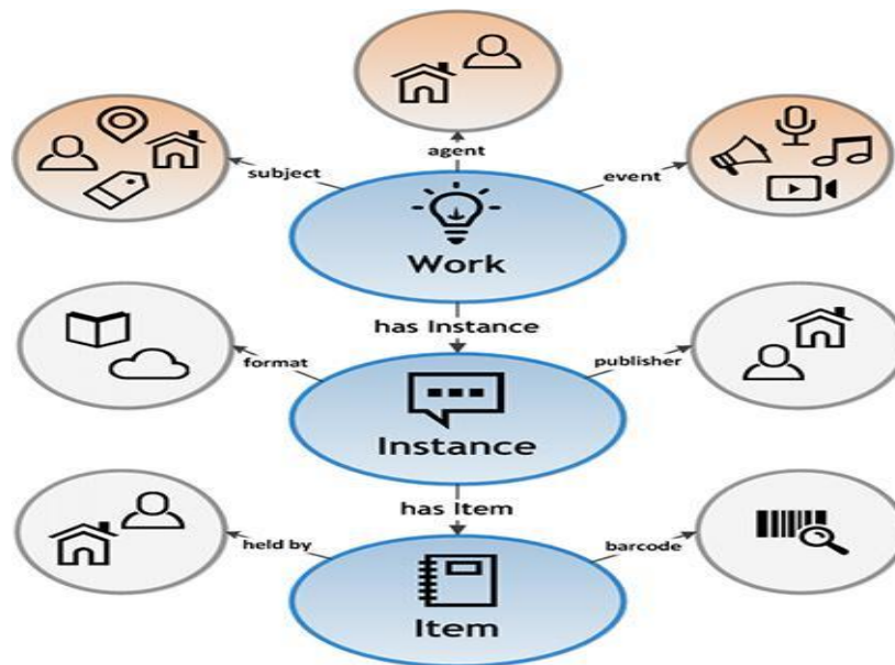
Σχ. 10 : Οι κλάσεις της οντολογίας BIBFRAME 2.0
