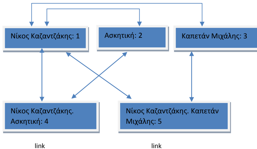
Σχ. 5: Standard τεχνική για την οντότητα Όνομα/Τίτλος
