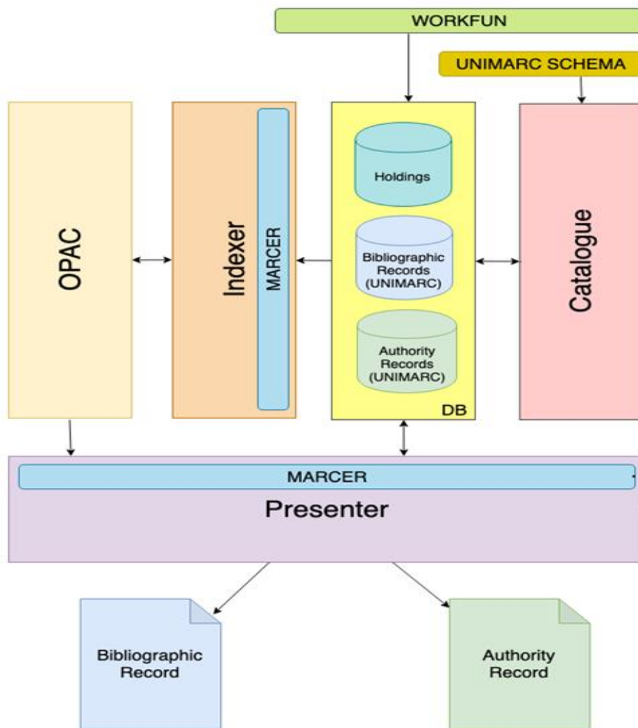
Σχ. 8: Αρχιτεκτονική συστήματος openABEKT
