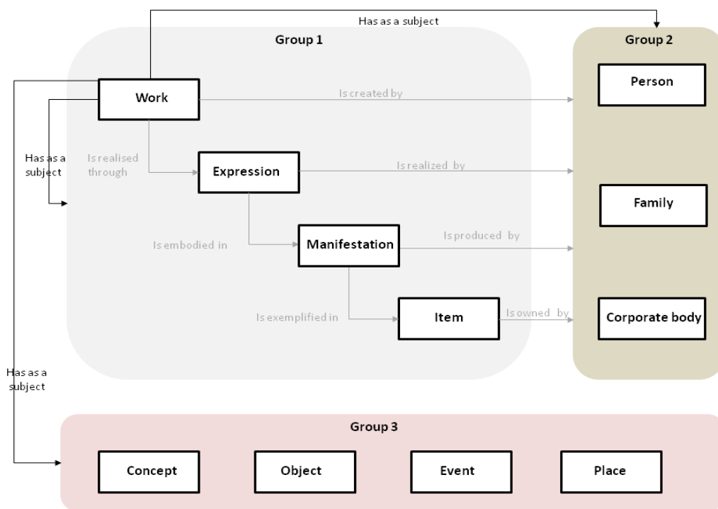
Σχ. 3: Οι FRBR ομάδες κλάσεων και οι βασικές σχέσεις μεταξύ τους
