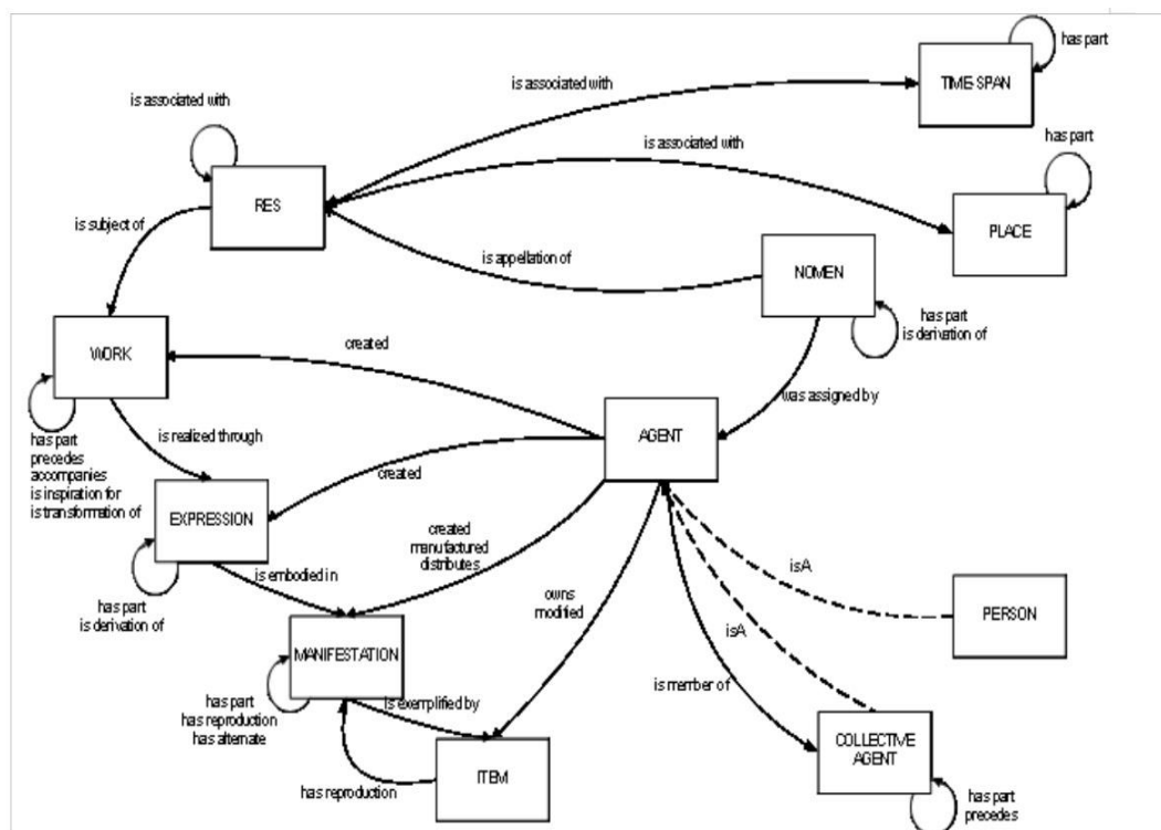
Σχ. 12 : Αναπαράσταση της οντολογίας LRM
