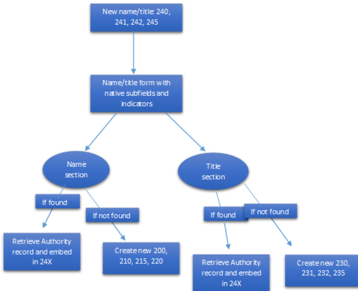
Σχ. 7: Η ροή εργασίας της δημιουργίας ενσωματωμένου Ονόματος/Τίτλου στο openABEKT
